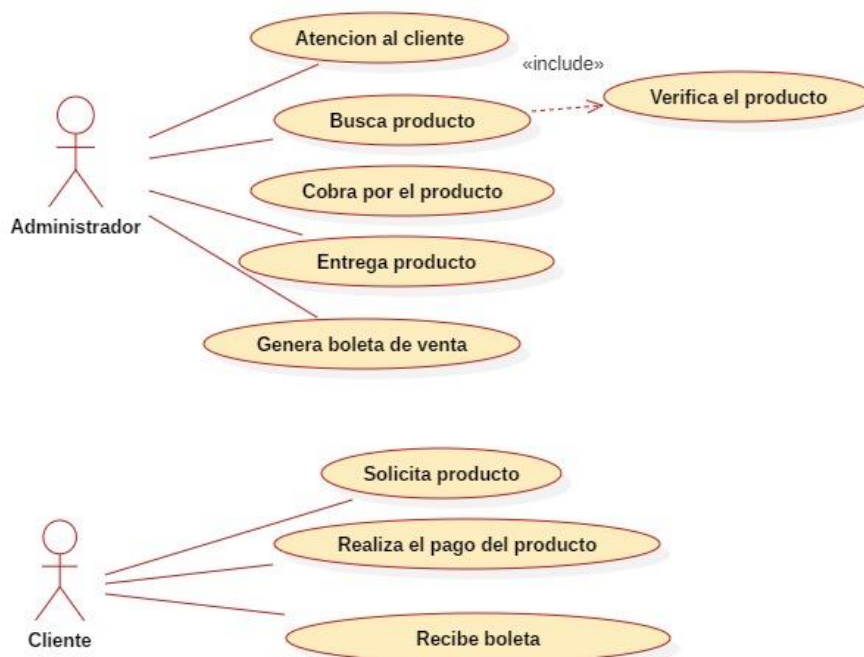
Figura 10: Análisis del proceso actual – Proceso de ventas de productos
