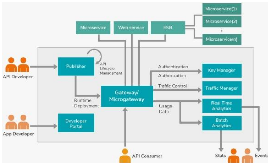
Figura 2: Funcionalidad del API's
