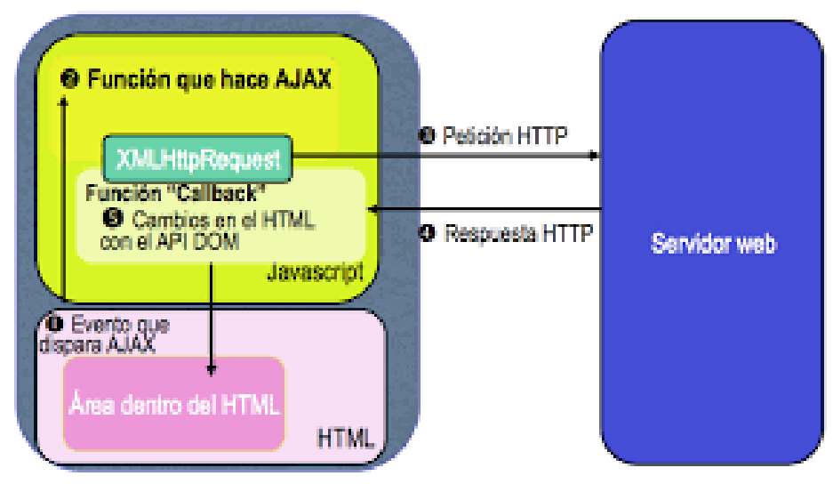
Figura 7: Concepto de Ajax
