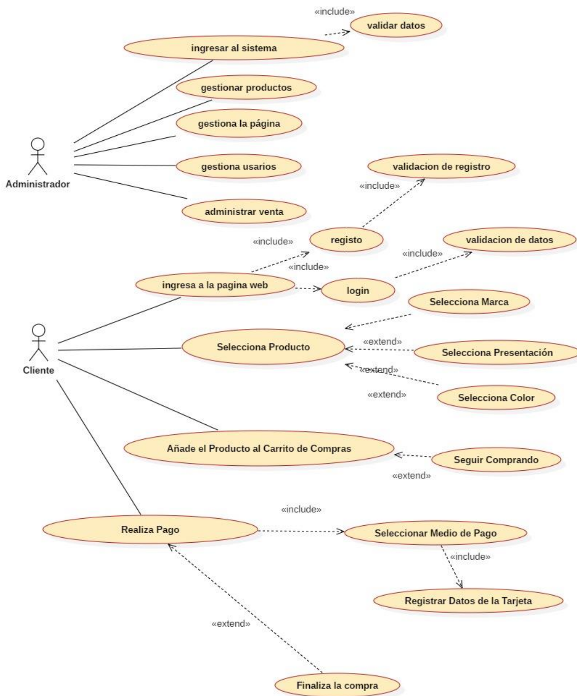
Figura 11: Análisis del proceso propuesto – Proceso de ventas de productos
